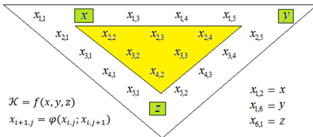
Рис. 5: Пример расположения аргументов функции в контуре массива
