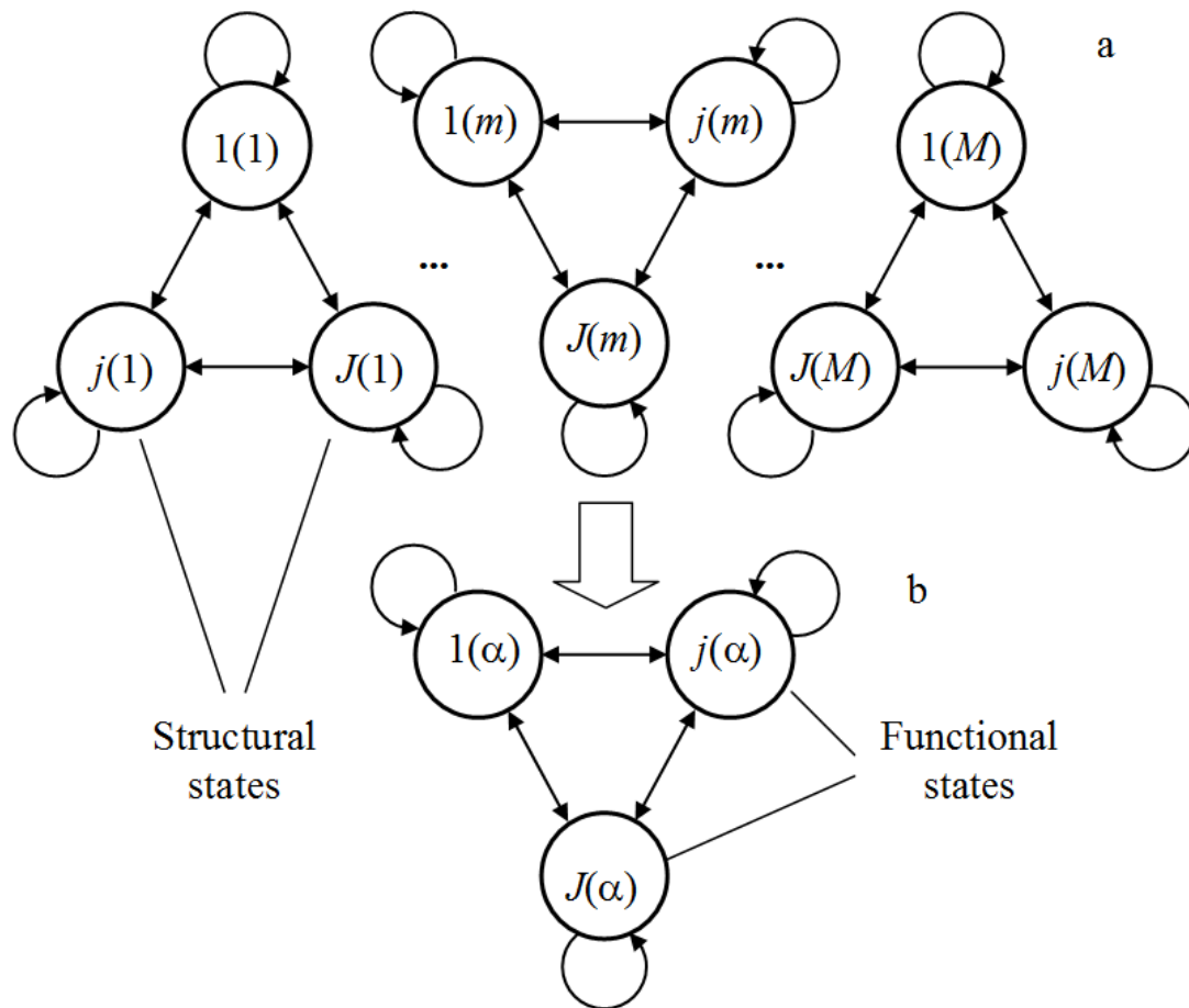
Рис. 2: Параллельный (а) и комплексный (б) полумарковские процессы
